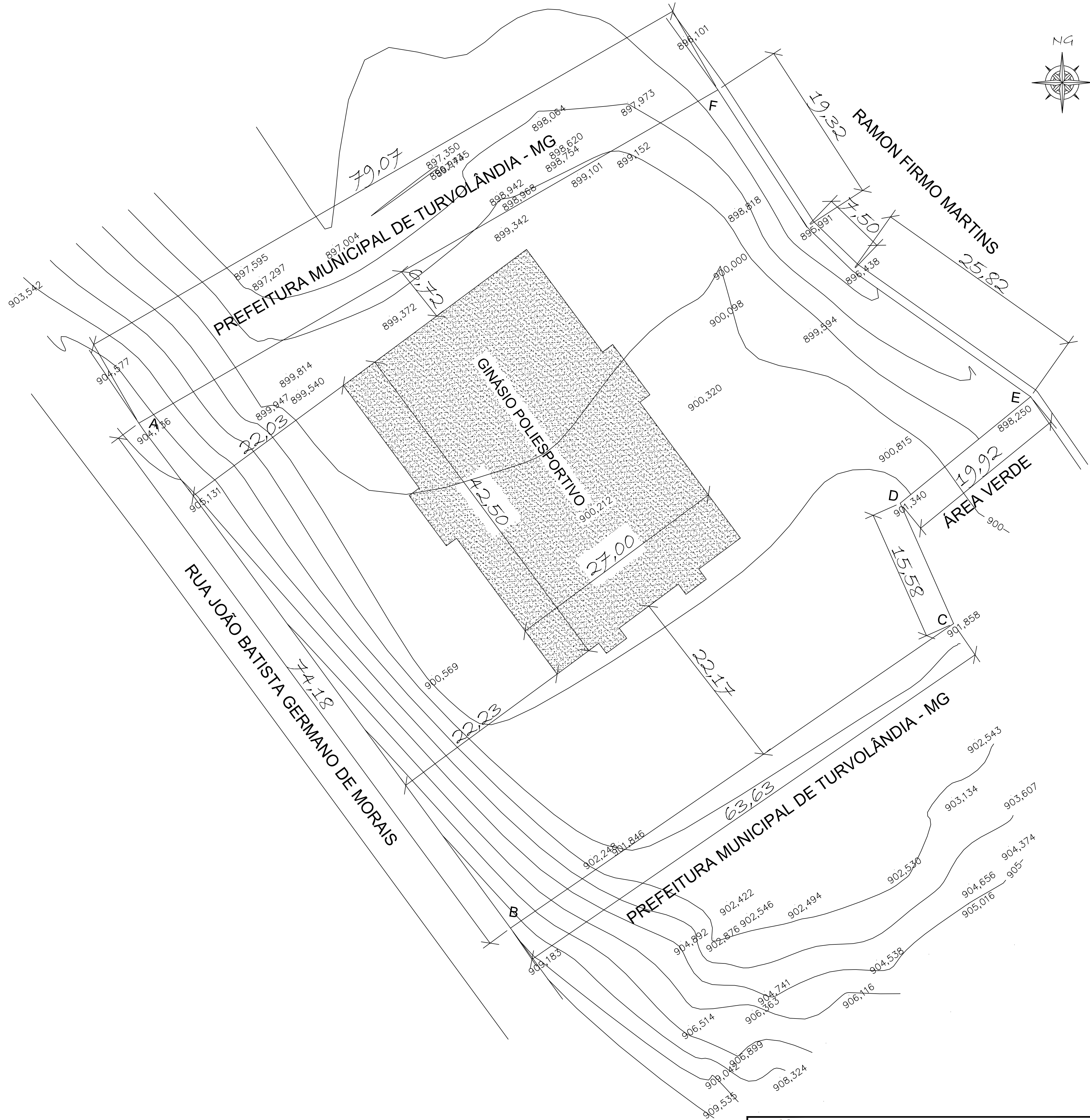
IMPLANTAÇÃO ESCALA 1/250
